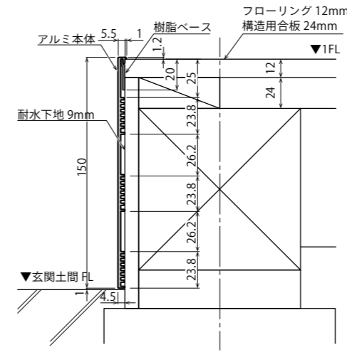
直線施工納まり (側面図・H150)
