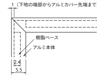
入隅コーナー部納まり (平面図・H150・50 共通)
