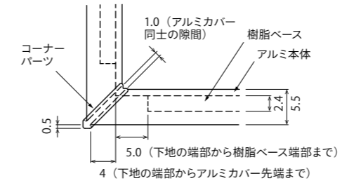
出隅コーナー部納まり (平面図・H150・50 共通)
